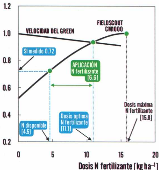
Figura 1 Modelos de respuesta de la calidad de juego (velocidad del green) y estética (FieldScout CM1000) a la dosis de N fertilizante en un green de Agrostis stolonifera en primavera. Los valores aparecen normalizados representando el índice de suficiencia [SI]. Ejemplo de cálculo del N que es necesario aplicar.
