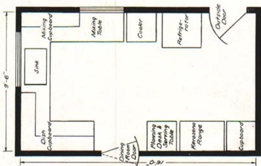
Fig. 28. Broken U-arrangement.
