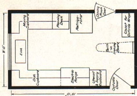
Fig. 27. U-arrangement.
